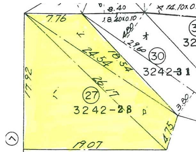
地積測量図
