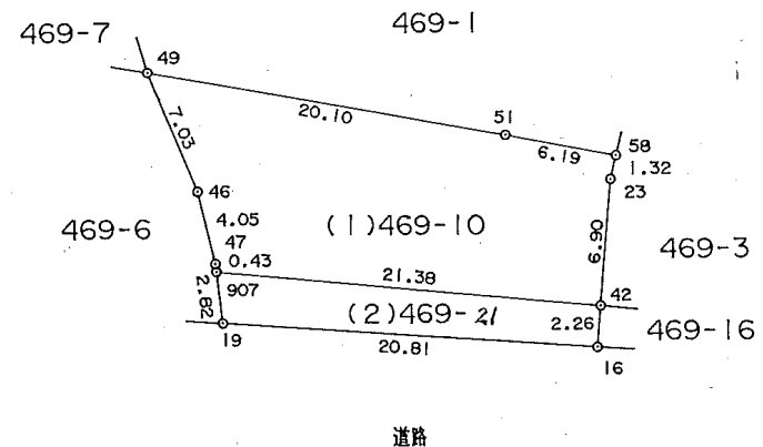
地積測量図
