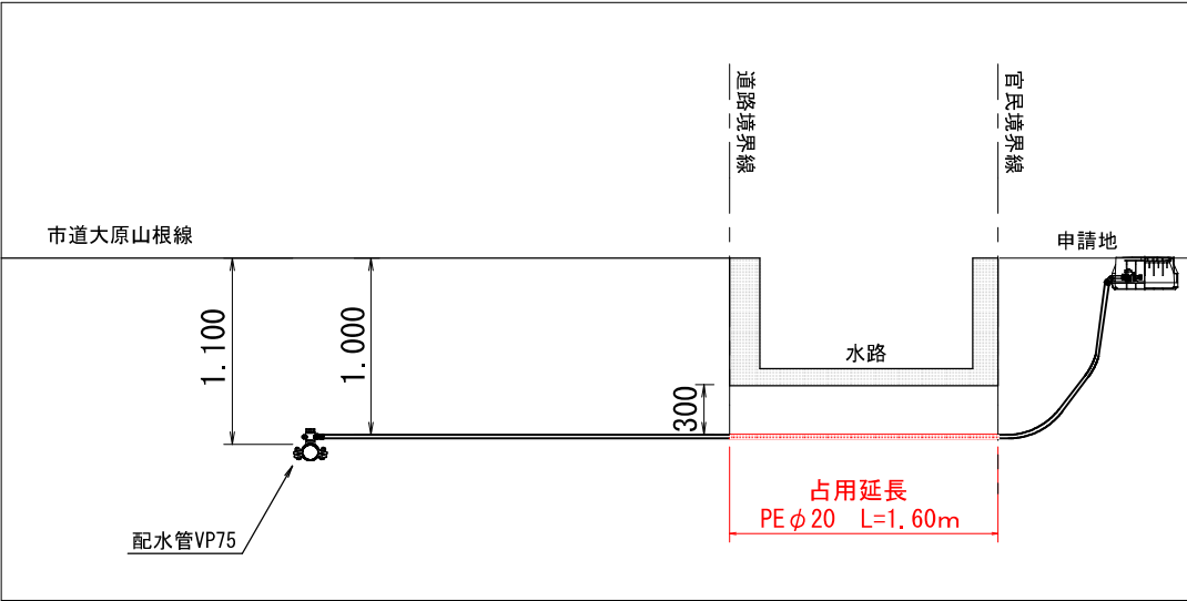
断面図 (S=1/50)
