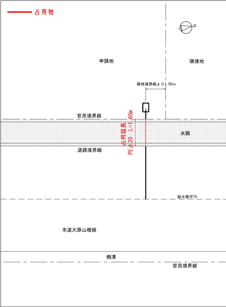
平面図 (S=1/100)
