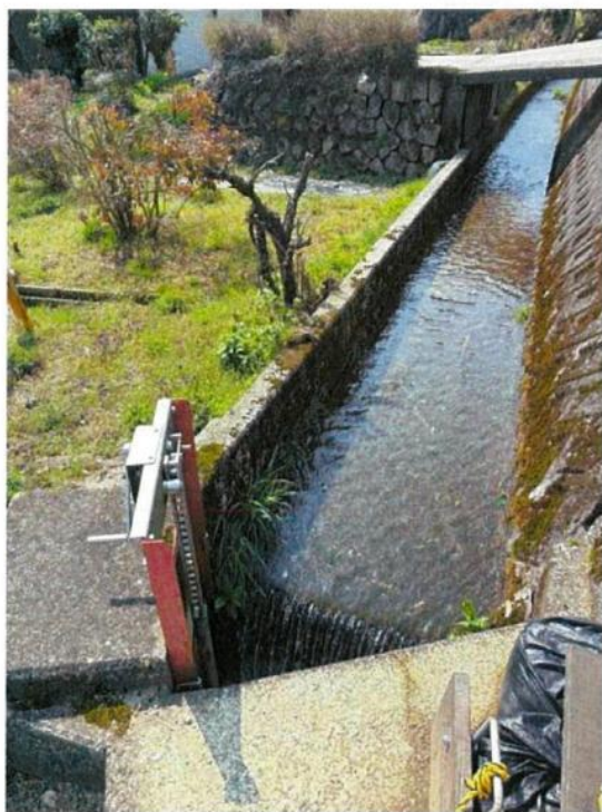
①用水路から余水吐ゲート
