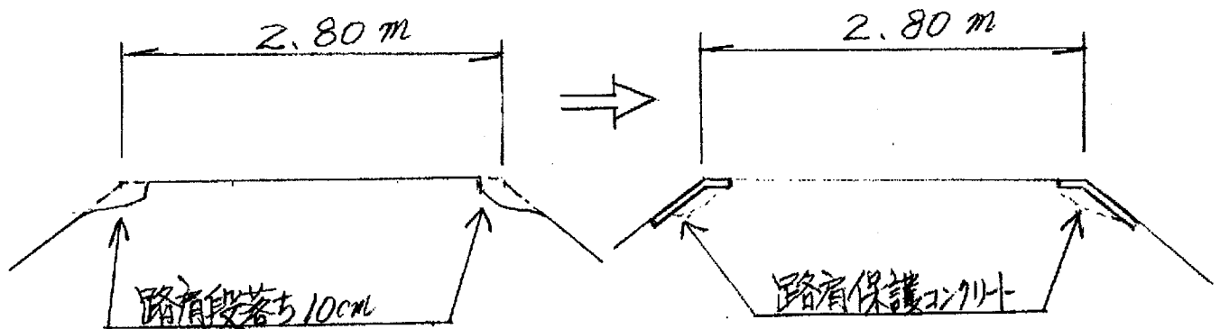
箇所番号 ①
