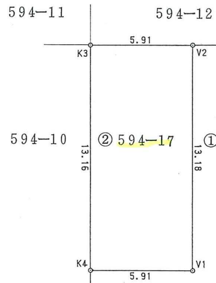
地積測量図
