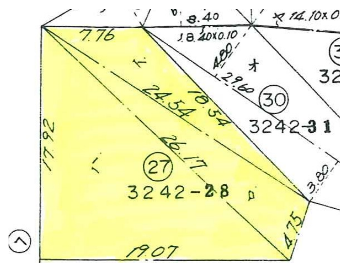
地積測量図
