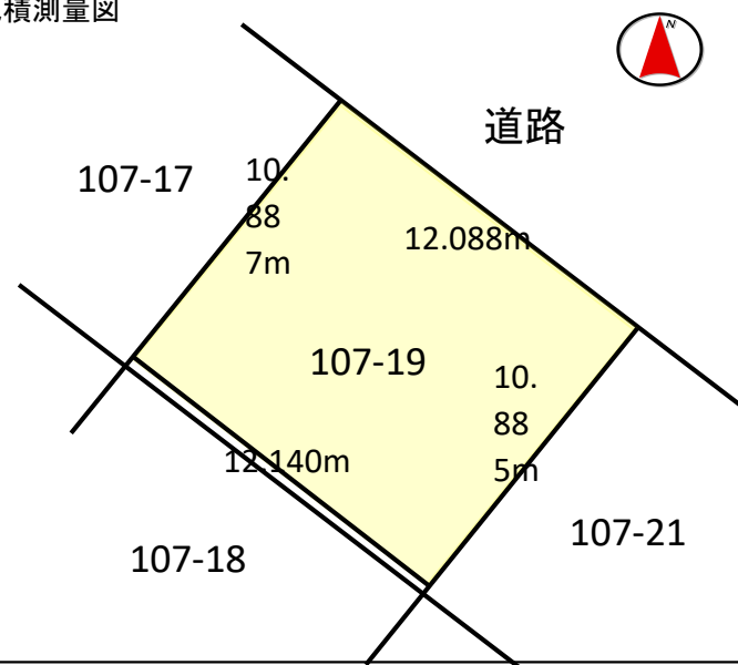
地積測量図
