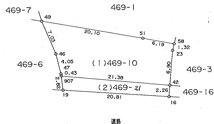
地積測量図
