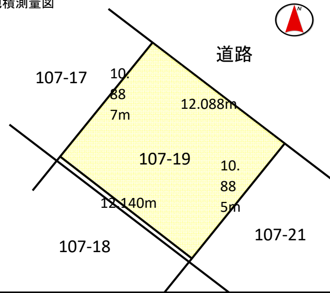
地積測量図
