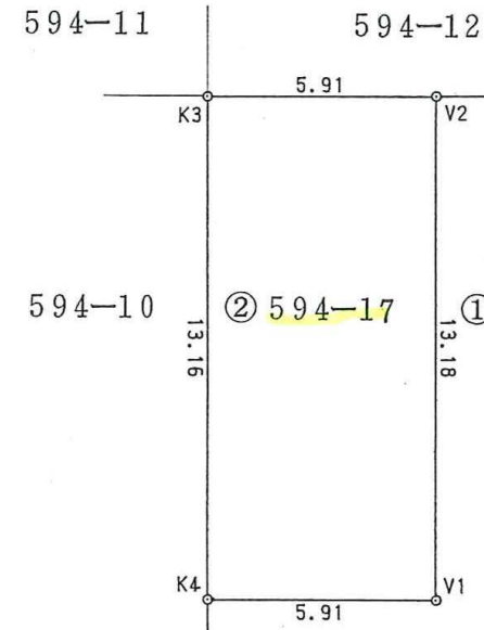
地積測量図
