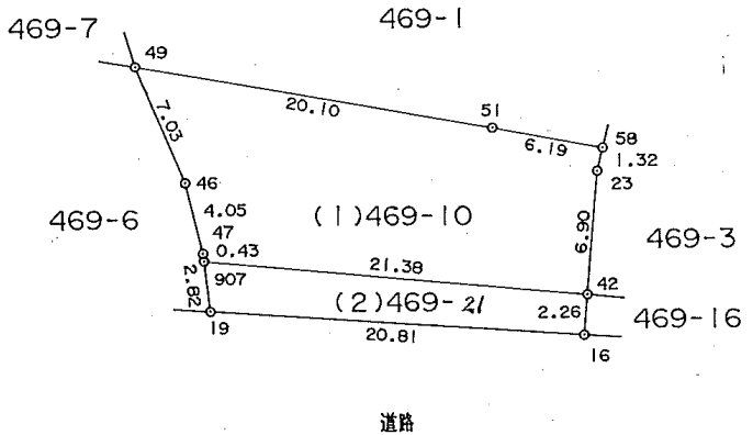
地積測量図
