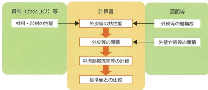
図 外皮計算の基本的な流れ
