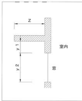
日除け寸法の取り方
