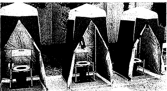
マンホールトイレ(長岡京市HP参照)
